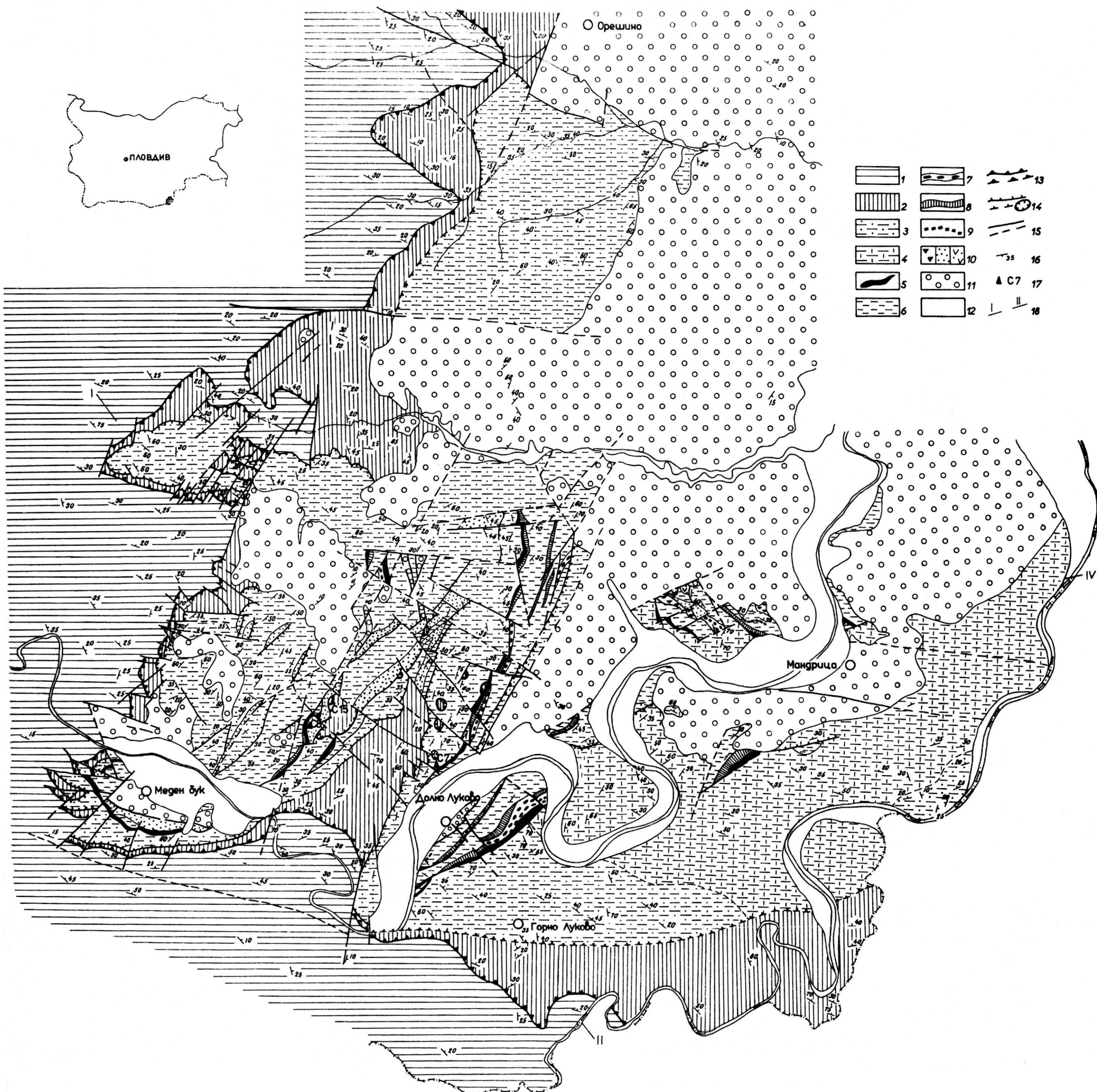
Рис. 11. Геологическая карта района Мандрица — Долно-Луково: 1 — параавтохтон — Прародопская надгруппа; 2 — аллохтон — Родопская надгруппа; Мандрицкая группа: 3 — Орешинская свита; 4 — Горнолуковская свита; Мигленицкая группа: 5 — Долнолуковская свита; 6 — кластолавовая пачка; 7 — олигостромовая пачка; 8 — конкреционная пачка; 9 — габбро-диабазы; Меденбукская свита; 10a — конгломерато-песчаниковая пачка; 10б — известковая песчаниково-туфогенная пачка;
