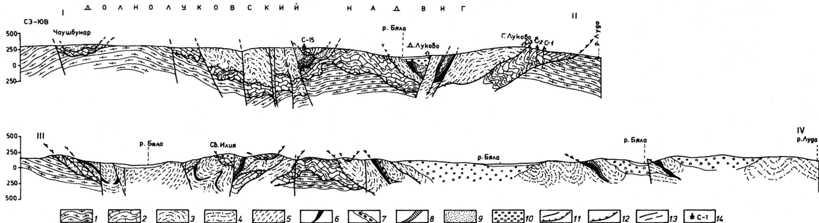
Рис. 12. Разрезы через фрагмент Восточнородопского комплексного надвига — Долнолуковский надвиг 1 — параавтохтон — Прародопская надгруппа; 2 — аллохтон — Родопская надгруппа; Мандрицкая группа; 3 — Орешниковская свита; 4 — Горнолуковская свита; Мыленицкая группа; 5 — Долнолуков-
